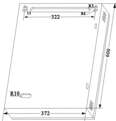
SSDH-J610R型电气火灾监控设备(壁挂式)安装图
